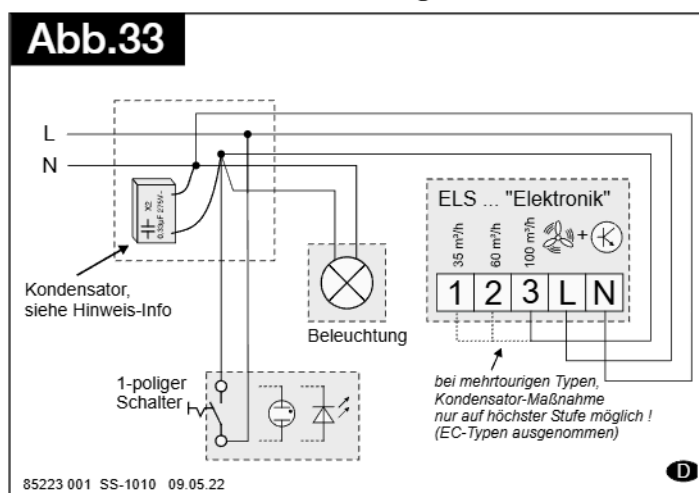
SS-1010 Lösung mit Kondensator
