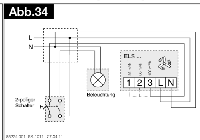
SS-1011 Lösung mit 2-poligem Schalter
