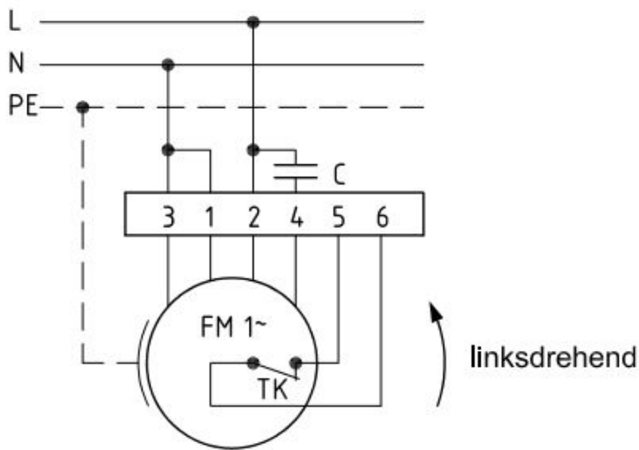
Anschlußplan 0.11-1 I.
