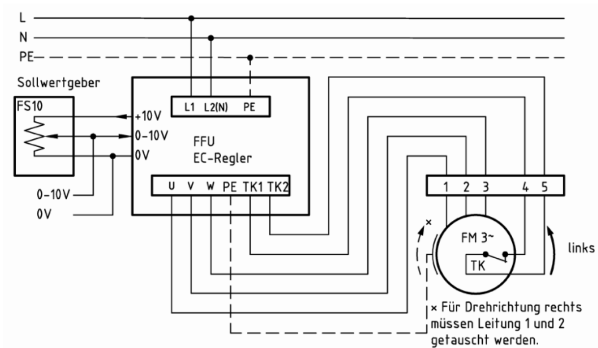
Anschlußplan FFU-EC 230
