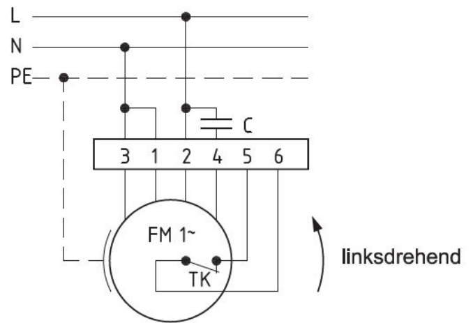
Anschlußplan 0.11-1 l.
