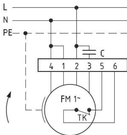
Anschlußplan 0.11-1 r.
