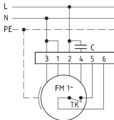
Anschlußplan 0.11-1 l.
