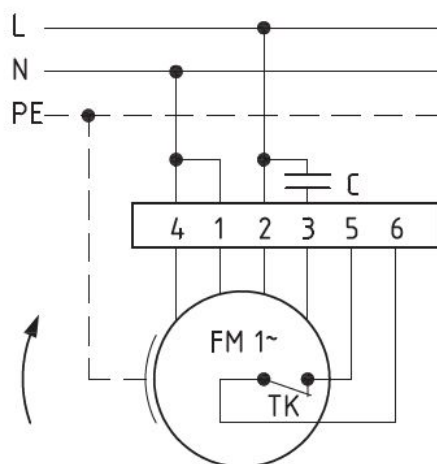
Anschlußplan 0.11-1 r.
