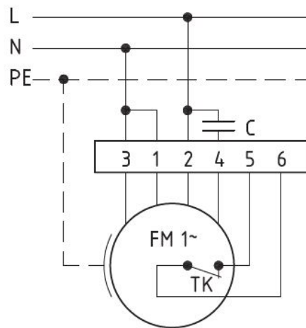
Anschlußplan 0.11-1 l.
