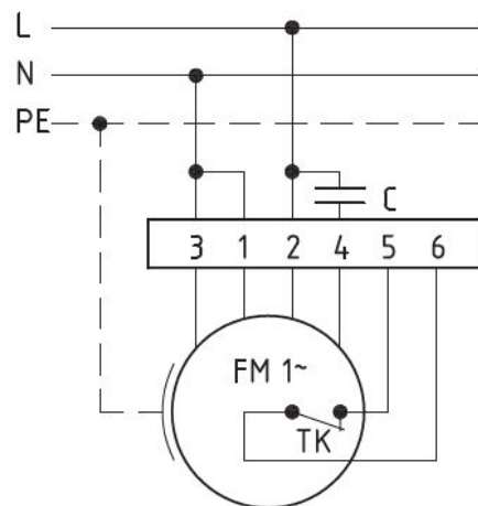
Anschlußplan 0.11-1 l.
