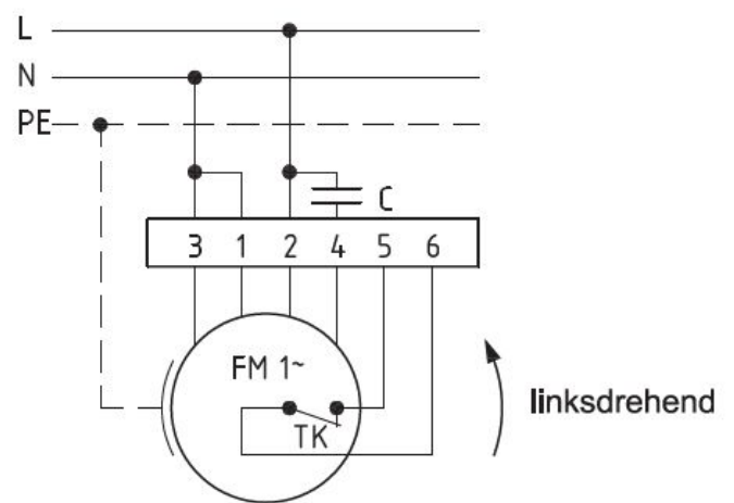
Anschlußplan 0.11-1 l.
