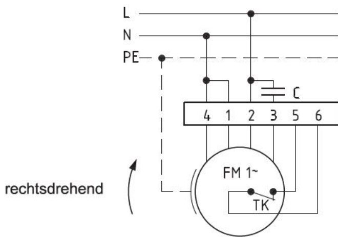
Anschlußplan 0.11-1 r.
