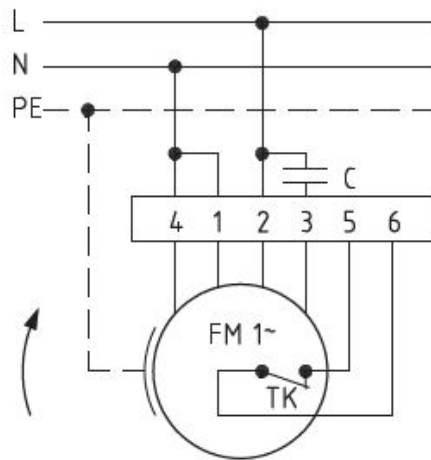
Anschlußplan 0.11-1 r.
