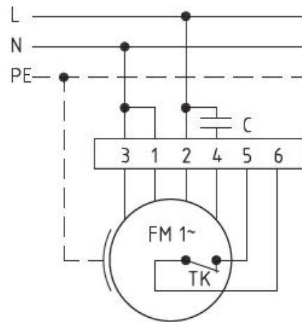
Anschlußplan 0.11-1 l.
