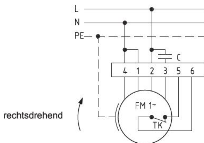
Anschlußplan 0.11-1 r.
