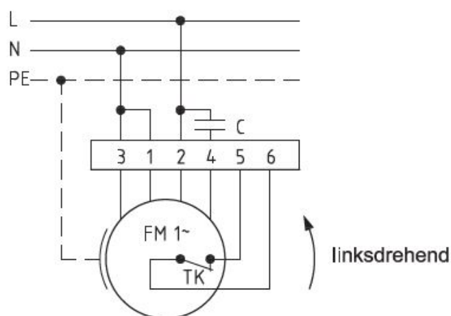
Anschlußplan 0.11-1 l.
