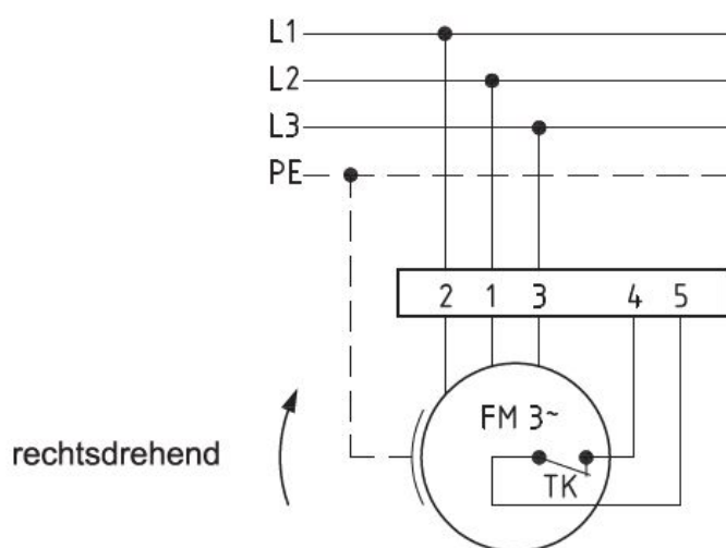
Anschlußplan 0.13-2 r.
