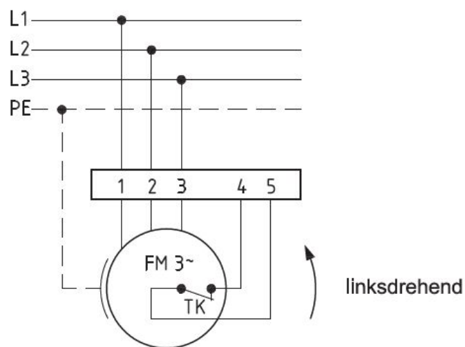
Anschlußplan 0.13-2 l.
