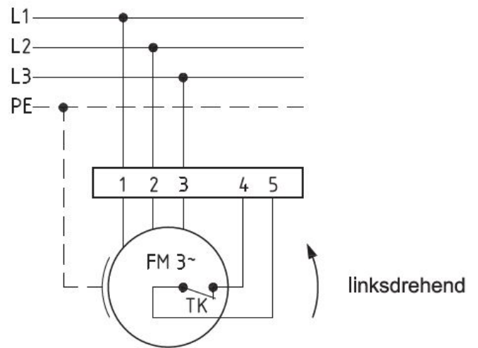
Anschlußplan 0.13-2 l.
