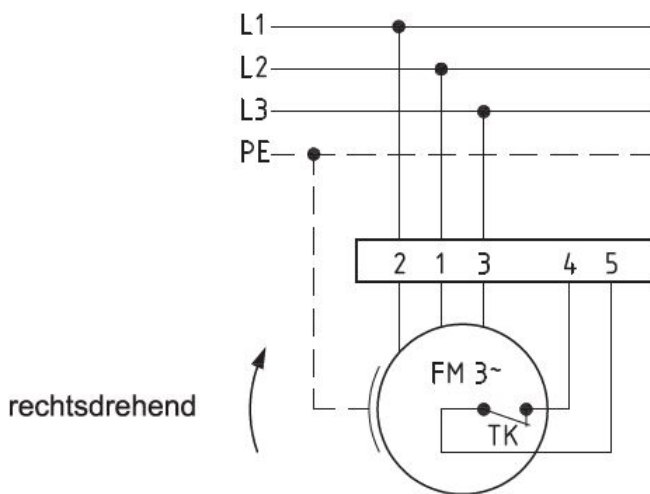
Anschlußplan 0.13-2 r.
