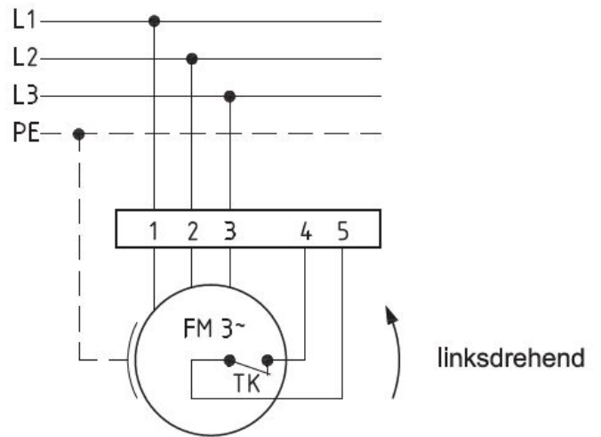
Anschlußplan 0.13-2 l.
