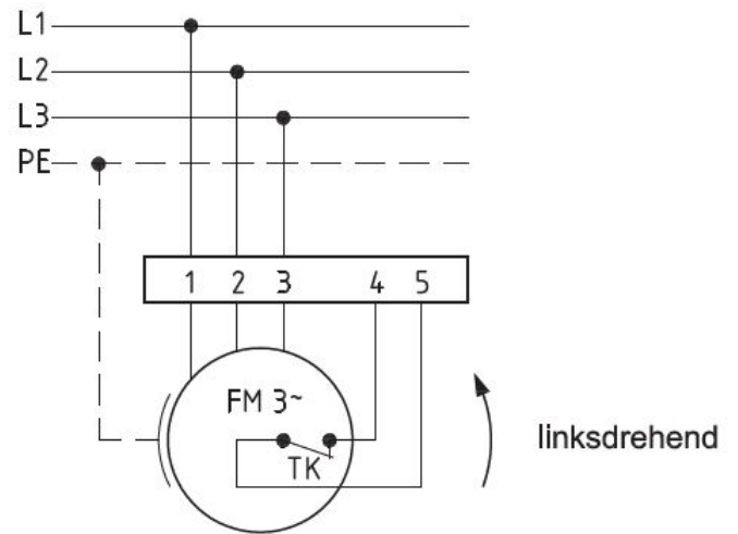
Anschlußplan 0.13-2 l.
