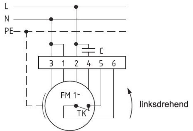
Anschlußplan 0.11-1 l.
