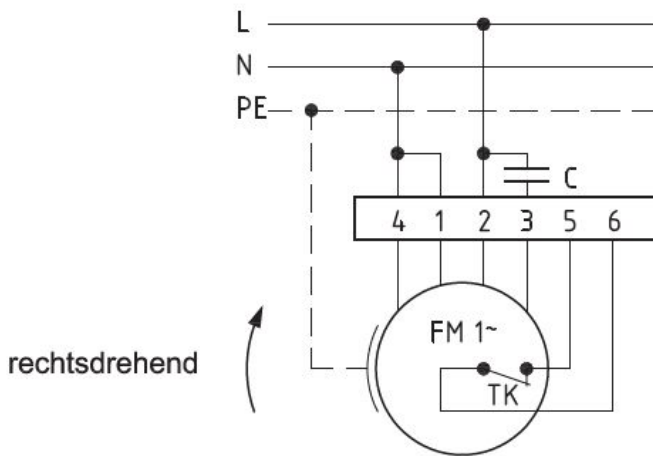
Anschlußplan 0.11-1 r.
