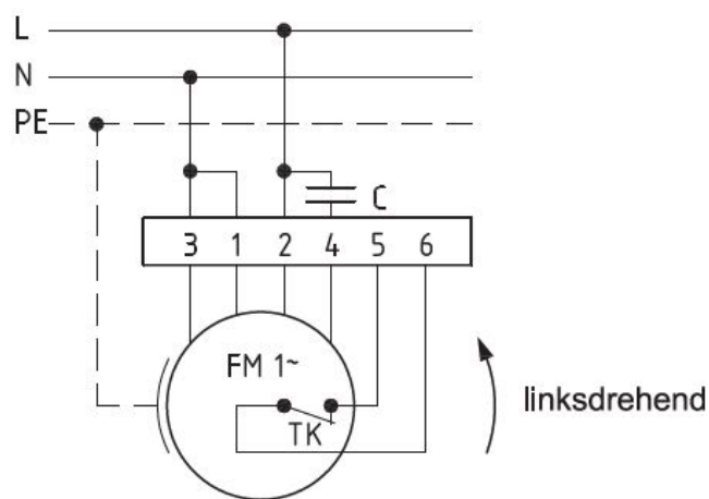
Anschlußplan 0.11-1 l.
