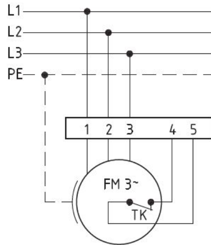
Anschlußplan 0.13-2 l.
