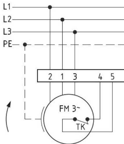
Anschlußplan 0.13-2 r.
