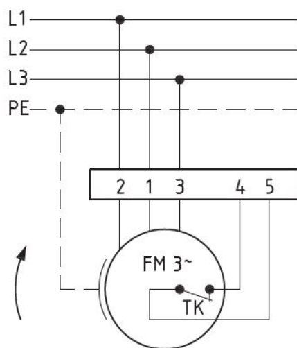
Anschlußplan 0.13-2 r.
