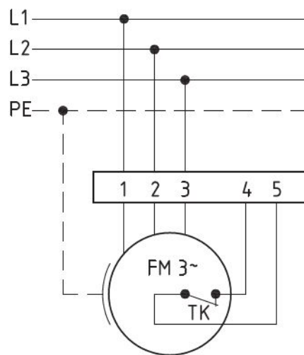
Anschlußplan 0.13-2 l.
