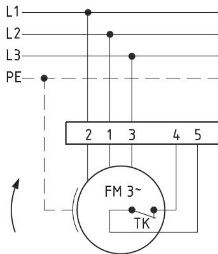
Anschlußplan 0.13-2 r.
