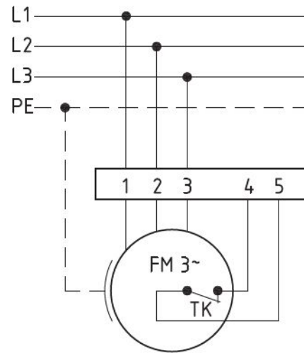
Anschlußplan 0.13-2 l.
