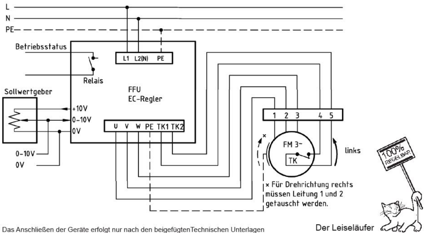
Anschlußplan* FFU-EC 230
