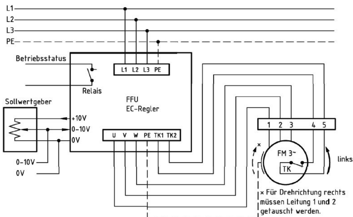
Anschlußplan* FFU-EC 400
