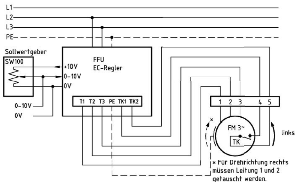
Anschlußplan FFU-EC
