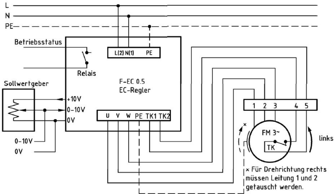
Anschlußplan F-EC 0.5
