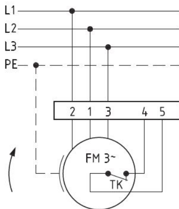
Anschlußplan 0.13-2 r.
