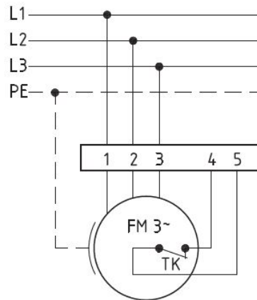
Anschlußplan 0.13-2 l.
