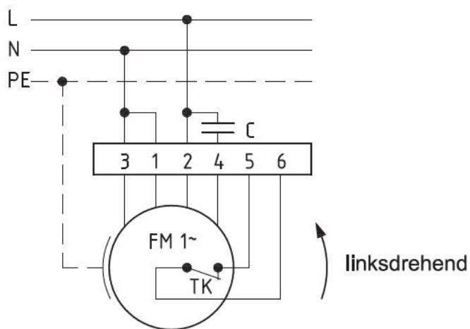
Anschlußplan 0.11-1 I.
