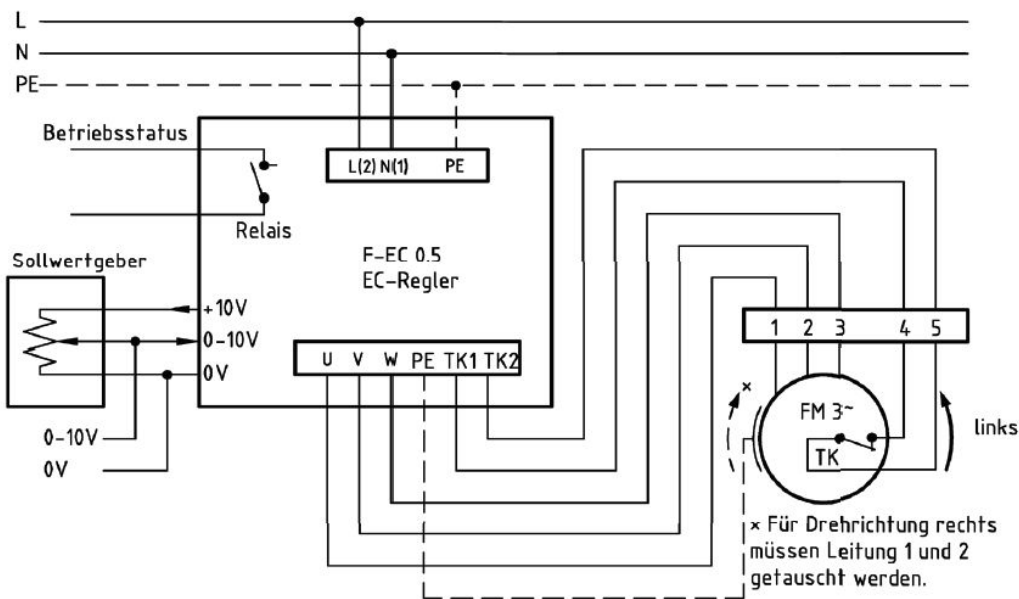
Anschlußplan F-EC 0.5
