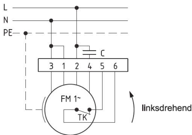
Anschlußplan 0.11-1 I.
