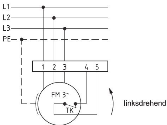
Anschlußplan 0.13-2 I.
