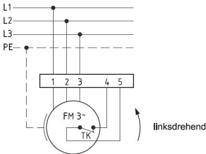
Anschlußplan 0.13-2 I.
