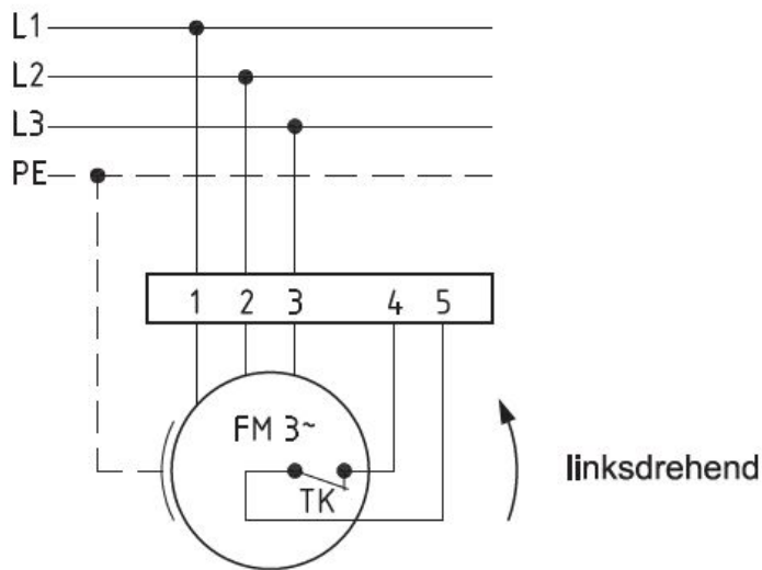
Anschlußplan 0.13-2 I.
