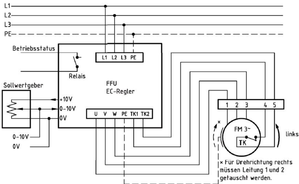
Anschlußplan FFU-EC 400
