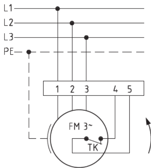
Anschlußplan 0.13-2 I.
