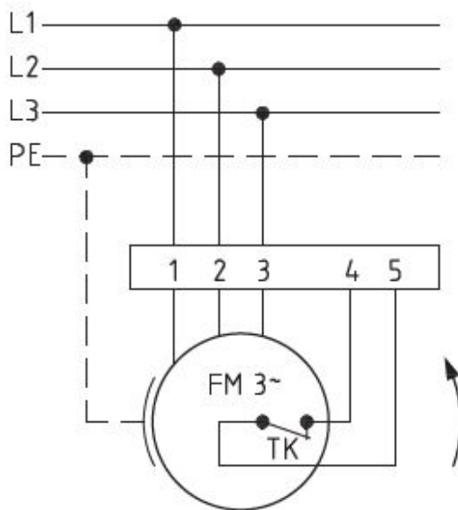
Anschlußplan 0.13-2 I.
