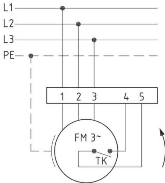
Anschlußplan 0.13-2 I.
