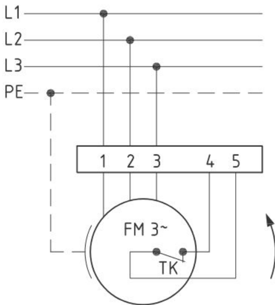
Anschlußplan 0.13-2 I.
