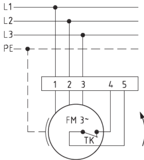
Anschlußplan 0.13-2 I.
