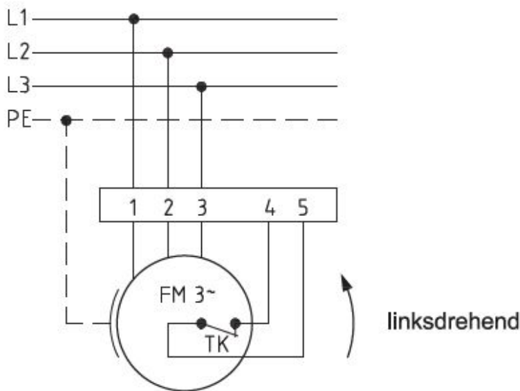
Anschlußplan 0.13-2 I.
