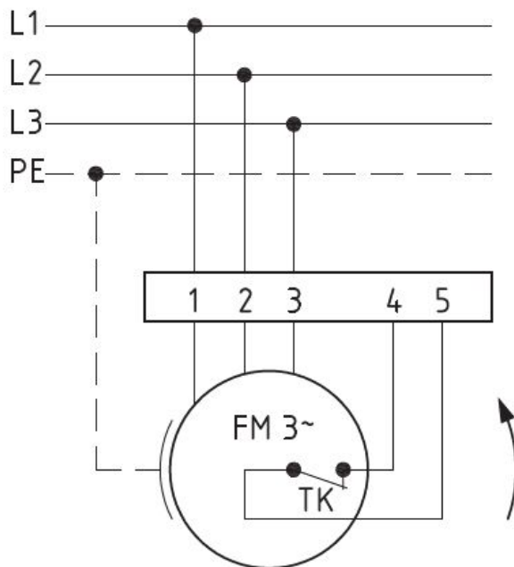
Anschlußplan 0.13-2 I.
