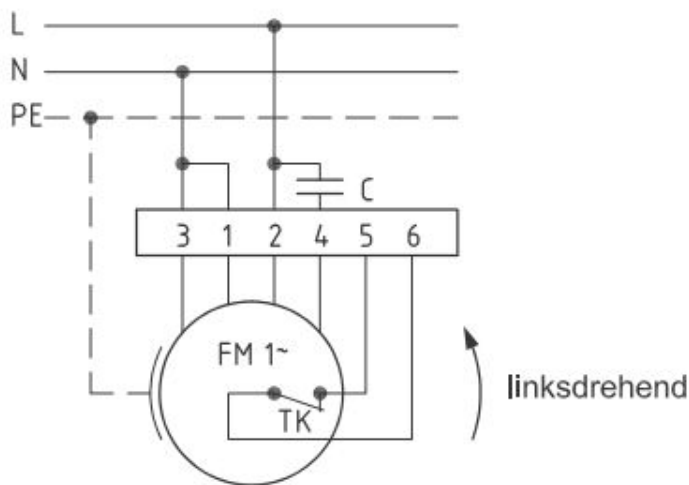
Anschlußplan 0.11-1 I.
