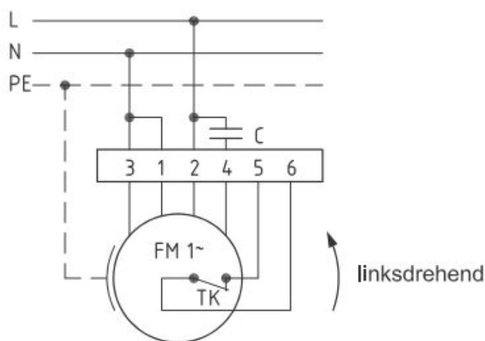
Anschlußplan 0.11-1 I.
