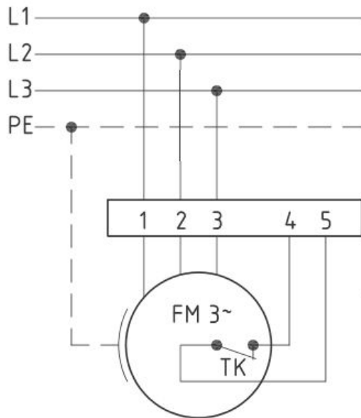
Anschlußplan 0.13-2 I.
