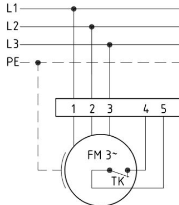
Anschlußplan 0.11-1 l.
