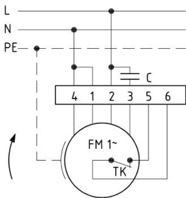
Anschlußplan 0.11-1 r.
