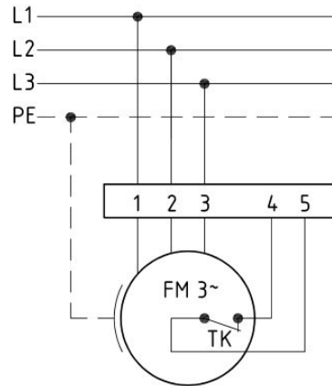
Anschlußplan 0.11-1 l.
