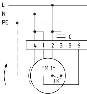
Anschlußplan 0.11-1 r.
