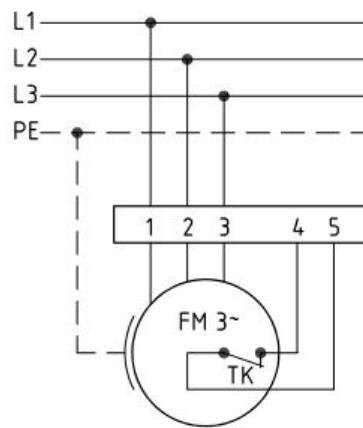
Anschlußplan 0.13-2 l.
