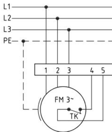
Anschlußplan 0.13-2 l.
