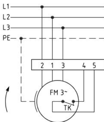
Anschlußplan 0.13-2 r.
