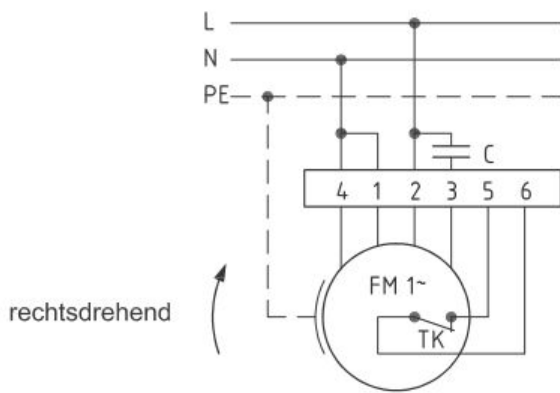
Anschlußplan 0.11-1 r.
