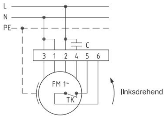
Anschlußplan 0.11-1 l.
