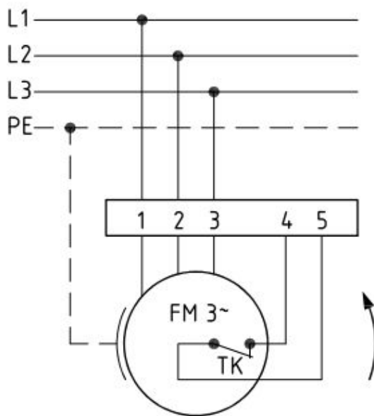
Anschlußplan 0.13-2 I.
