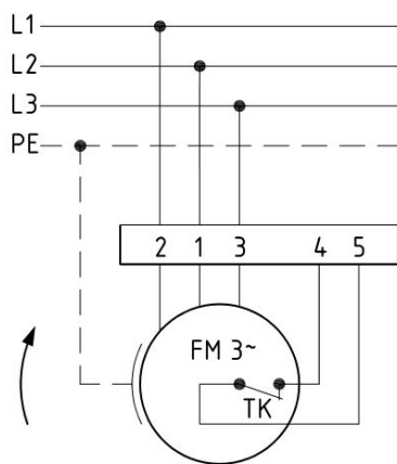
Anschlußplan 0.13-2 r.
