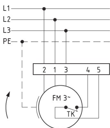
Anschlußplan 0.13-2 r.
