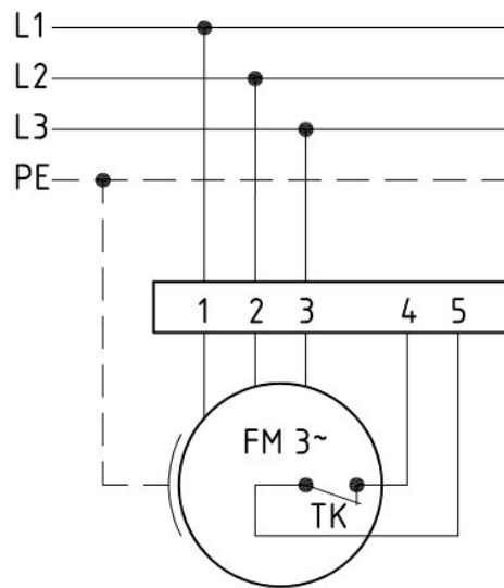
Anschlußplan 0.13-2 I.
